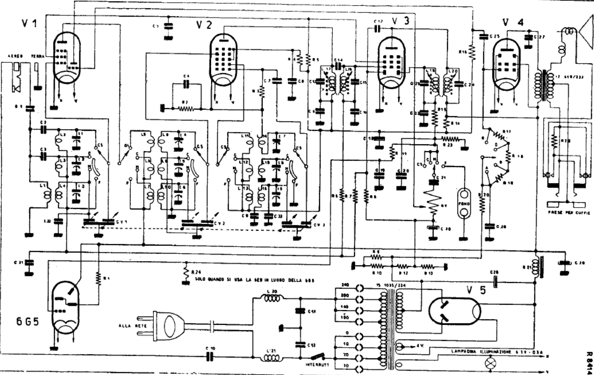
PHONOLA (S. A. FIMI). — Mod. 559/F. — Media frequenza: 470 kHz. VALVOLE: V1 = 6P7G; V2 = 6A8G; V3 = 6BN8G; V4 = 6V6G; V5 = 5Y3G.
